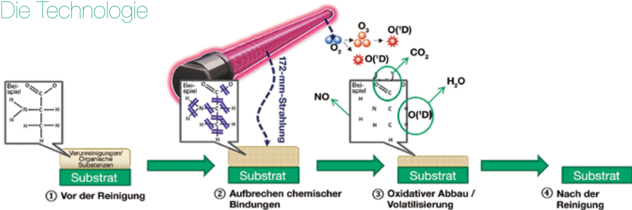
Excimer-Prinzip
